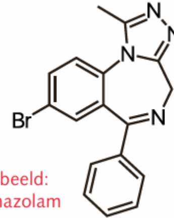
Voorbeeld: pyrazolam
